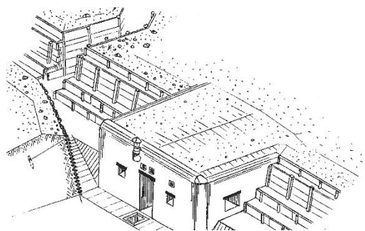
Vue générale d'un abri de piquet de garde dans une tranchée de première ligne. P. Burtscher « de la ceinture fortifiée de Strasbourg à la position de la Bruche »
